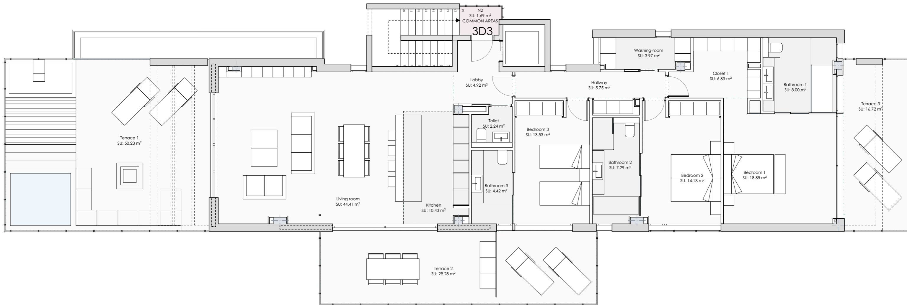
2 -PENTHOUSE
