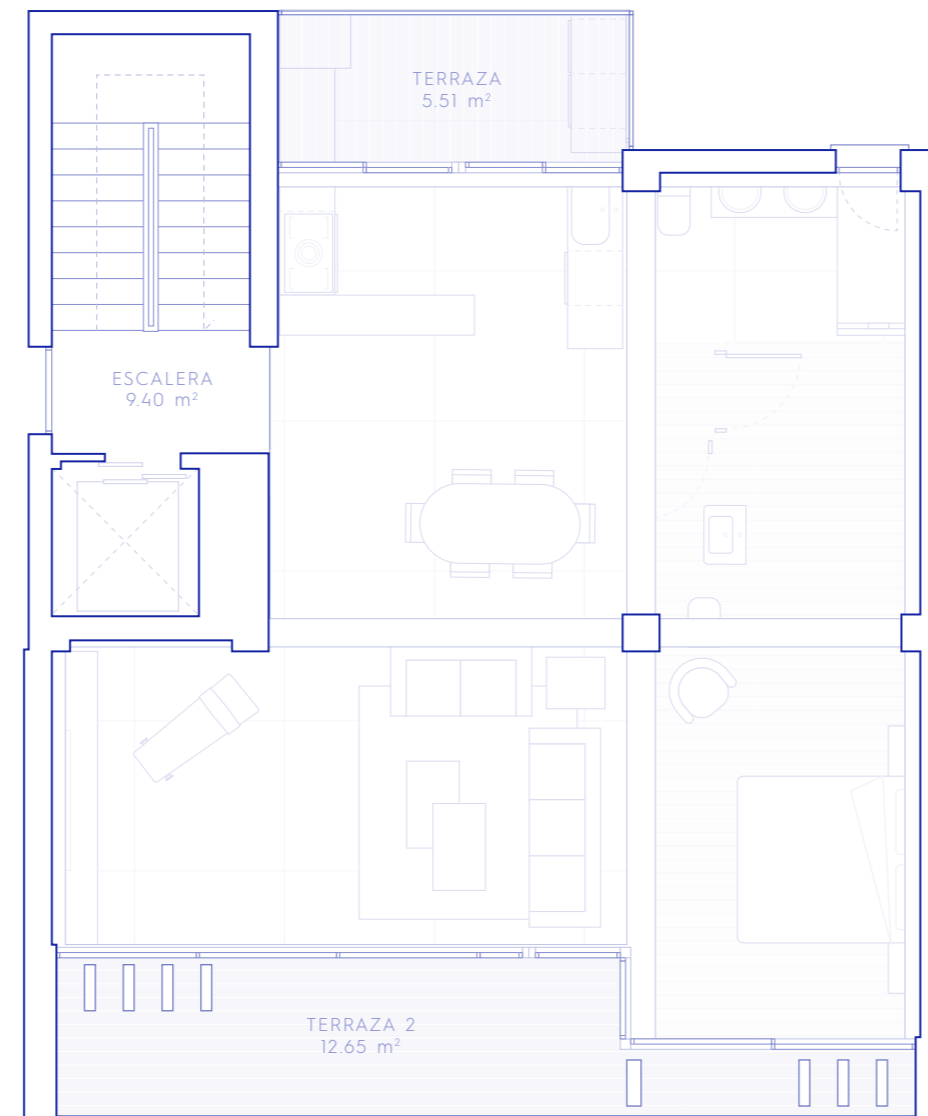
PLANTA SEGUNDA
